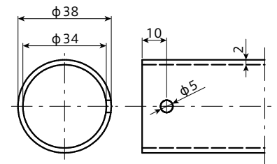
製品図 SUS304
